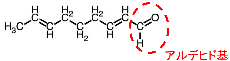
ノナジエナール
