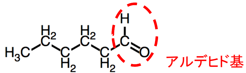
ヘキサナール
